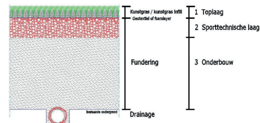
Figuur 2.1 Opbouw van een kunstgrasveld Onderstaand lichten we de drie onderdelen van een kunstgrasveld (toplaag, sporttechnische laag en onderbouw) kort toe.
